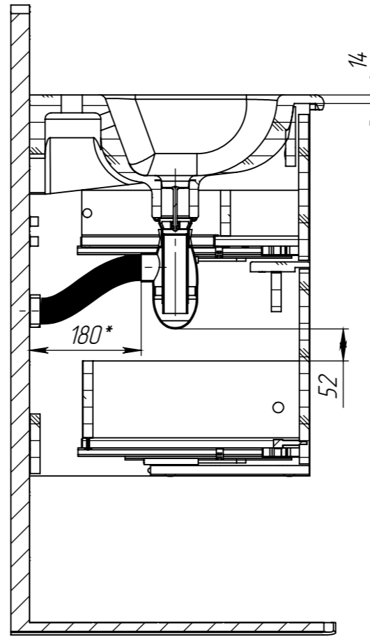
Уровень пола
